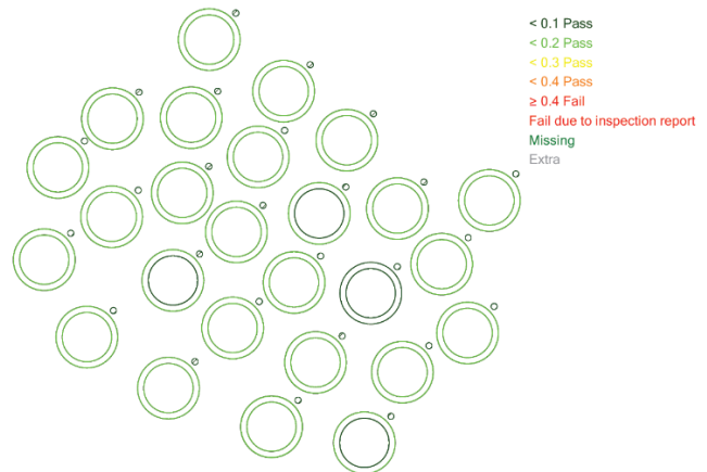
Abweichungskarte
